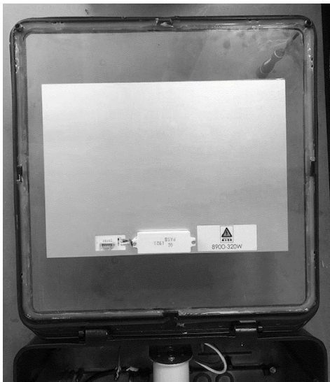
Figura 3 - Panel LED adherido al interior de la lente de vidrio
