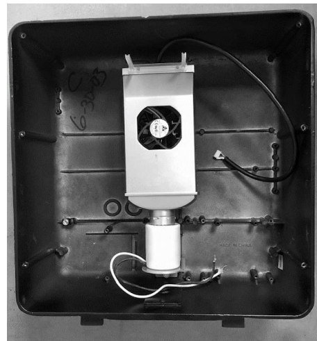
Figure 2 - Ballast contourné et retiré, pilote de mise à niveau LED installé avec des pieds de support
