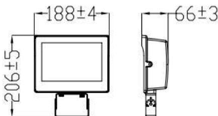
Trunion*
