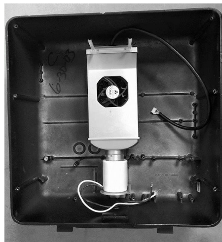
Figure 2 - Ballast contourné et retiré, pilote de mise à niveau LED installé avec des pieds de support
