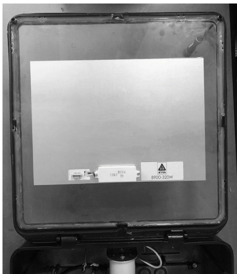
Figure 3 - Panneau LED collé à l'intérieur de la lentille en verre
