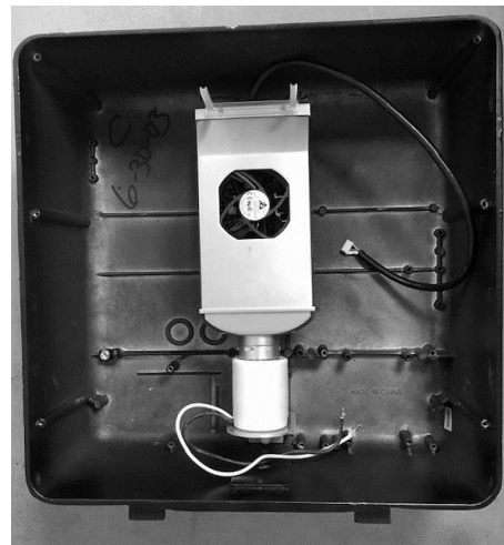
Figura 2 - Lastre puenteado y eliminado, controlador de actualización LED instalado con patas de soporte
