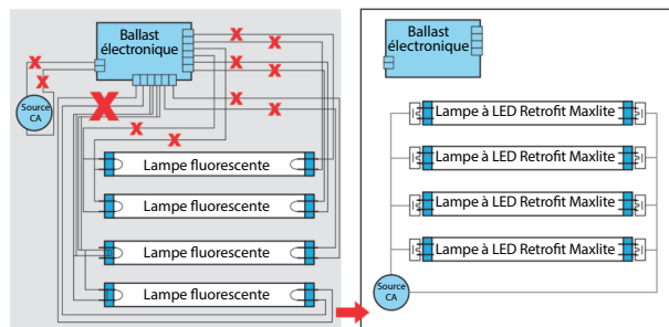
Figure 4. - Modernisation avec trois / quatre lampes
