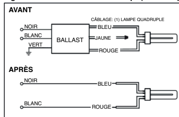
Figure 3. Modernisation avec une lampe (Base G24q)
