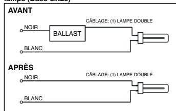
Figure 1. Modernisation avec une lampe (Base GX23)
