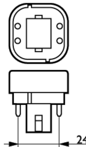
Base G24q-2
