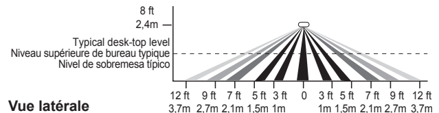
Vue latérale
