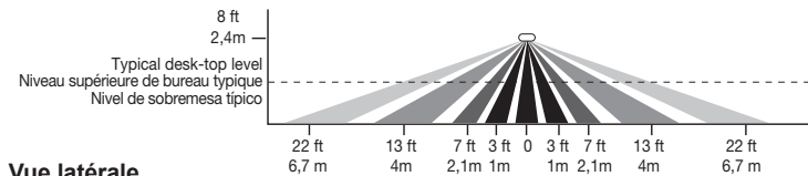
Vue latérale
