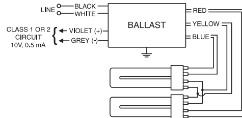
Diag. 59A
