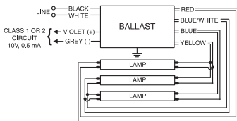
Diag. 57A
