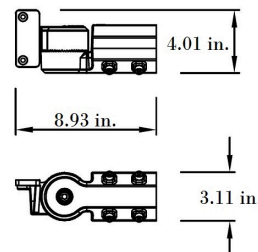
Slipfitter
