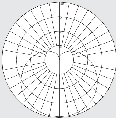
Nombre maximum de candelas : 118 Situé à angle horizontal = 67,5; angle vertical = 2,5 Plan vertical via angles horizontaux (250-80)
