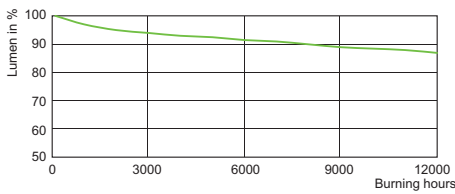
CDM-Rm 50W /930
