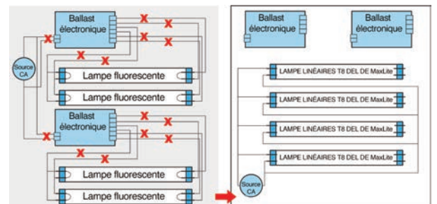
Figure 6. - Installation avec trois/quatre lampes et deux ballasts
