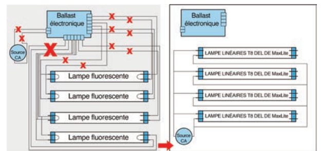
Figure 5. - Installation avec trois/quatre lampes
