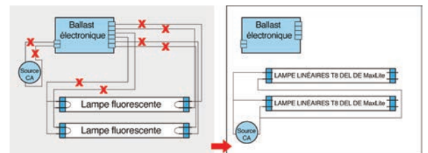
Figure 4. - Installation avec deux lampes
