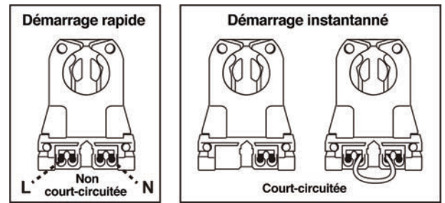
Figure 1. - Douilles non court-circuitée et court-circuitées
