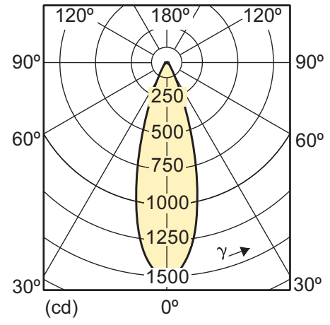
11-60W E26 3000K PAR30L 36D
