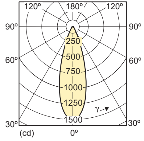
11-60W E26 2700K PAR30L 36D
