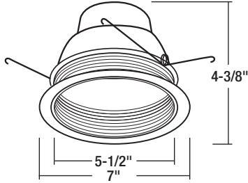
Trim OD: 7" Aperture: 5-1/2" Height: 4-3/8"
