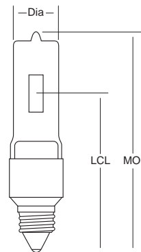
E11 Base
