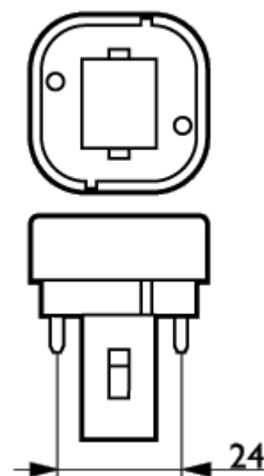
Base G24d-3
